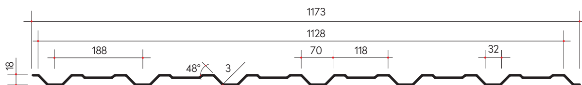
Trapecinis lakštas T-18FS / 1173 mm
