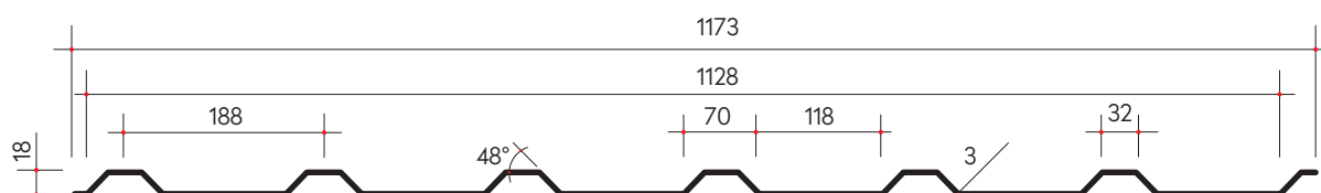
Trapecinis lakštas T-18S / 1173 mm
