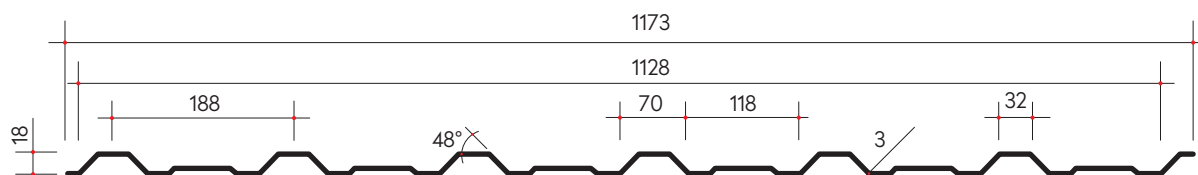
Trapecinis lakštas T-18SS / 1173 mm
