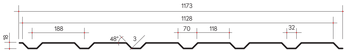
Trapecinis lakštas T-18F / 1173 mm
